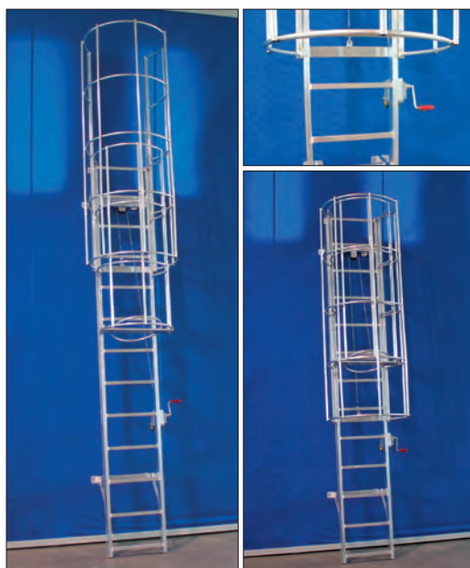
GABBIA TELESCOPICA CON ARGANO TELESCOPIC CAGE WITH WINCH
