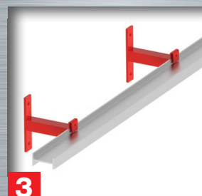
Staffe distanziatrici per fissaggio binario Spacer brackets for track fixing
